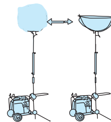
【台車付 LEDバルーン投光機 円筒or全光バルーン】
