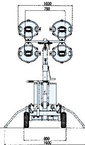
LB430F
